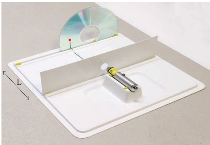
צילום 4 של מערכת הניסוי עם התקליטור, L = 10 cm
