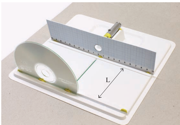
צילום 5 של מערכת הניסוי עם התקליטור, L = 10 cm
